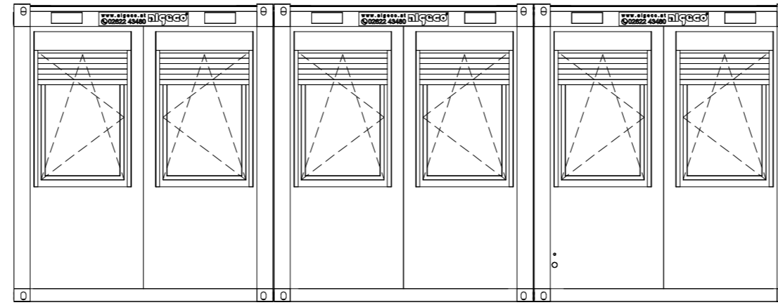
Ansicht Ost
